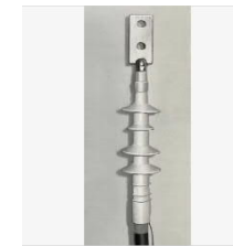
ĐẦU CÁP CO NGUỘI TRUNG THỂ TRONG NHÀ 36KV (Tr 21-22)
